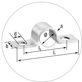
NORMAFIX® TYP BSL 512 PRO 1 TRUBKA (podle normy DIN 72573)
