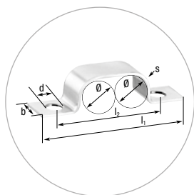
NORMAFIX® TYP BSL 512 PRO 2 TRUBKY (podle normy DIN 72573)
