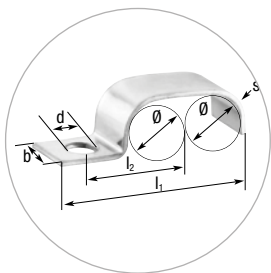
NORMAFIX® TYP BSL 510 PRO 2 TRUBKY (podle normy DIN 72571)
