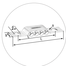
NORMAFIX® TYP BSL 512 PRO 4 TRUBKY (podle normy DIN 72573)
