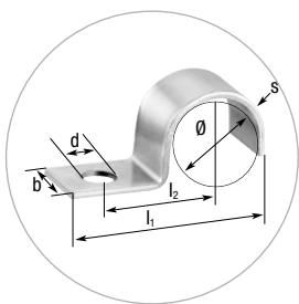
NORMAFIX® TYP BSL 510 PRO 1 TRUBKA (podle normy DIN 72571)
