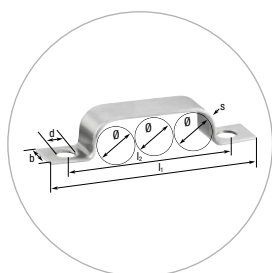
NORMAFIX® TYP BSL 512 PRO 3 TRUBKY (podle normy DIN 72573)
